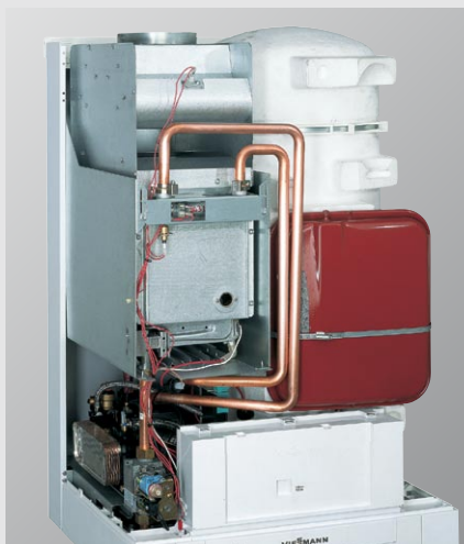
Vitopend 222-W – kompaktowy kocioł grzewczy ze zintegrowanym zasobnikiem c.w.u.
