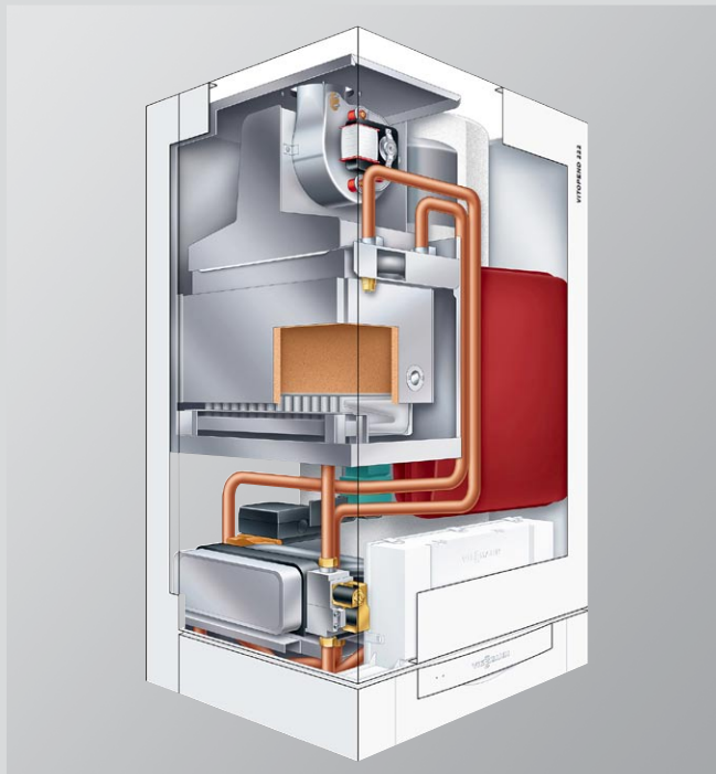
Vitopend 222-W 10,5 do 24 kW (30 kW w trybie „booster”)
