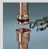
System połączeń wtykowych Multi-Steck.
